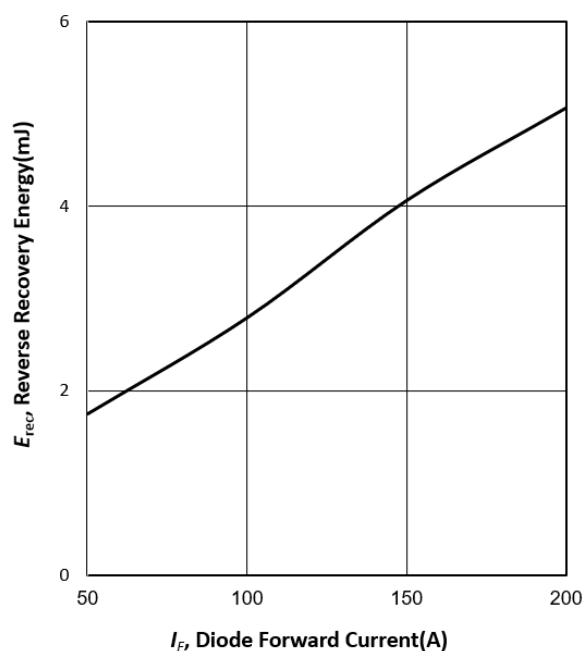
图 6 二极管反向恢复损耗与正向电流的关系 ( T_{vj}=25^{\circ}\text{C} , V_{CE}=600\text{V} , R_G=7.5\Omega )
