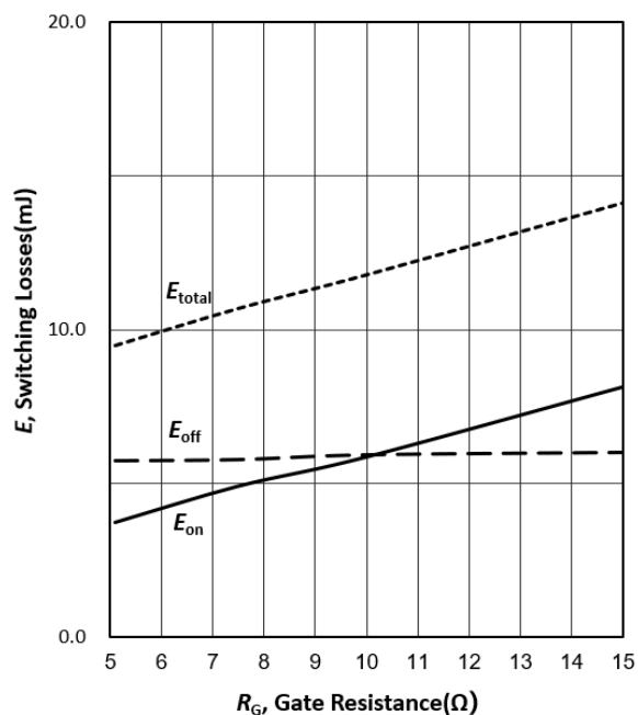
图 5 IGBT 开关损耗与栅极电阻的关系 (感性负载, T_{vj}=25^{\circ}\text{C} , V_{CE}=600\text{V} , V_{GE}=-15/15\text{V} , I_C=100\text{A} )
