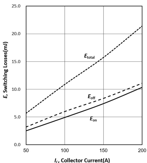
图 3 IGBT 开关损耗与集电极电流的关系 (感性负载, T_{vj}=25^{\circ}\text{C} , V_{CE}=600\text{V} , V_{GE}=-15/15\text{V} , R_G=7.5\ \Omega )
