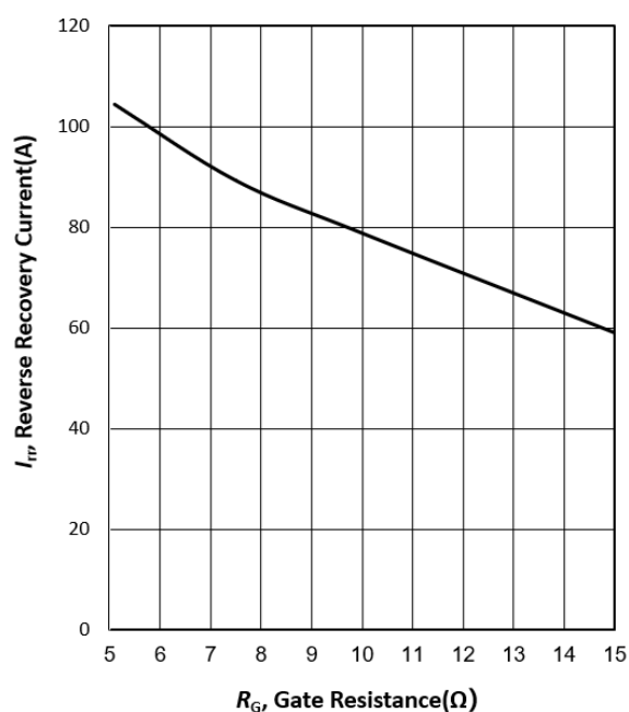
图 8 二极管反向恢复峰值电流与栅电阻的关系 ( T_{vj}=25^{\circ}\text{C} , V_{CE}=600\text{V} , I_F=100\text{A} )
