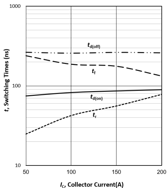
图 2 IGBT 开关时间与集电极电流的关系 (感性负载, T_{vj}=25^{\circ}\text{C} , V_{CE}=600\text{V} , V_{GE}=-15/15\text{V} , R_G=7.5\ \Omega )
