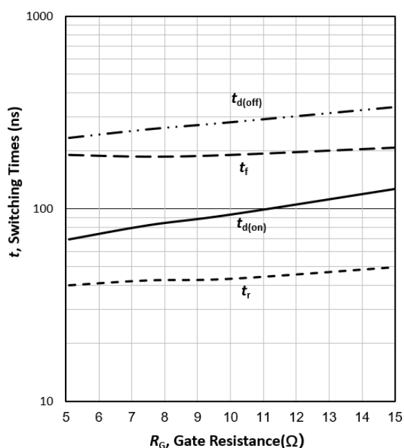
图 4 IGBT 开关时间与栅极电阻的关系 (感性负载, T_{vj}=25^{\circ}\text{C} , V_{CE}=600\text{V} , V_{GE}=-15/15\text{V} , I_C=100\text{A} )
