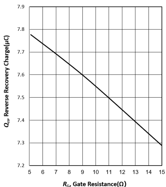
图 7 二极管反向恢复电荷与栅电阻的关系 ( T_{vj}=25^{\circ}\text{C} , V_{CE}=600\text{V} , I_F=100\text{A} )
