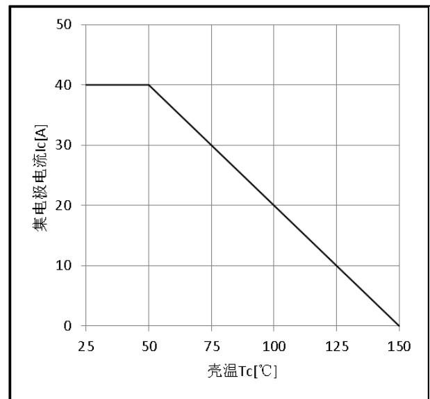
图 16 集电极电流温度特性
