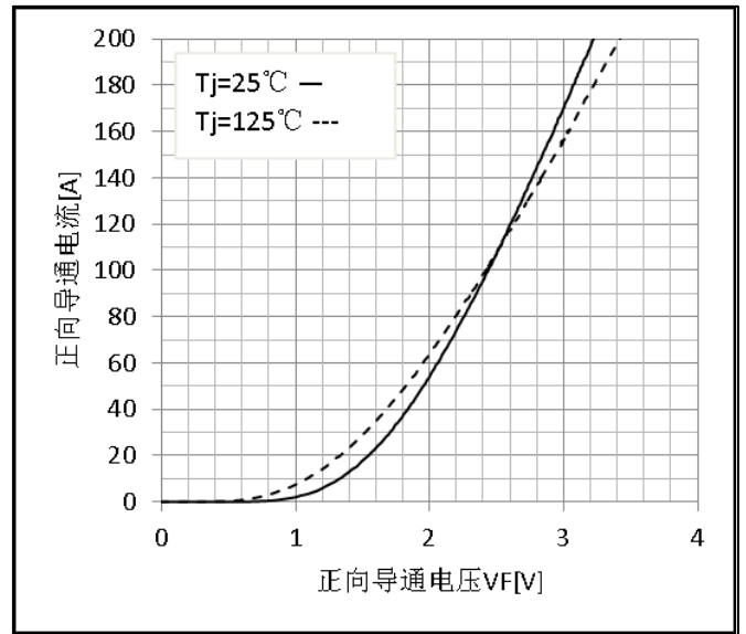
图 18 二极管正向特性
