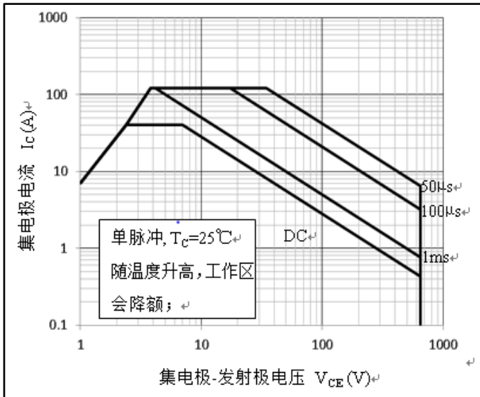
图 17 正偏安全工作区
