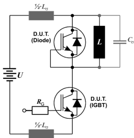
图 E 开关参数测试电路
