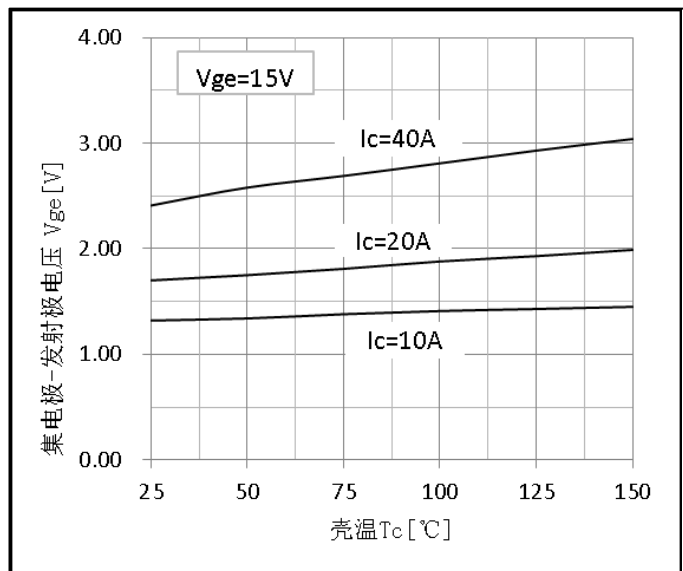
图 4 饱和压降温度特性
