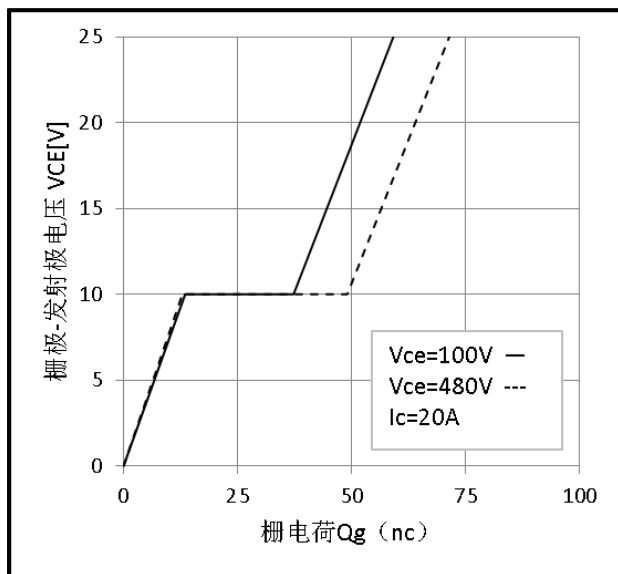
图 15 栅电荷特性
