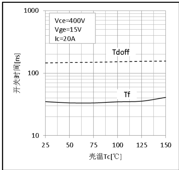
图 9 关断时间与壳温的关系 (感性负载, 测试电路参考图 E)
