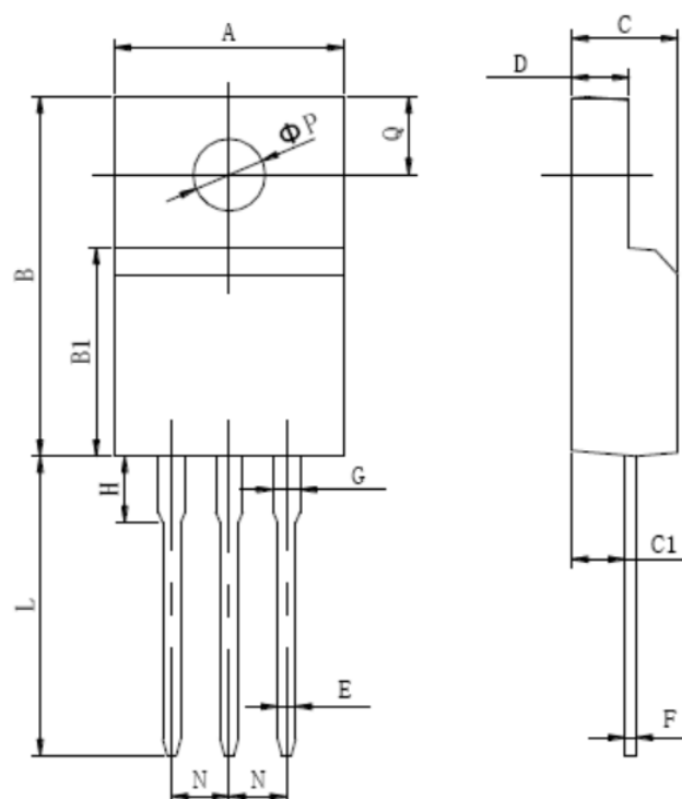
TO-220 封装尺寸图
