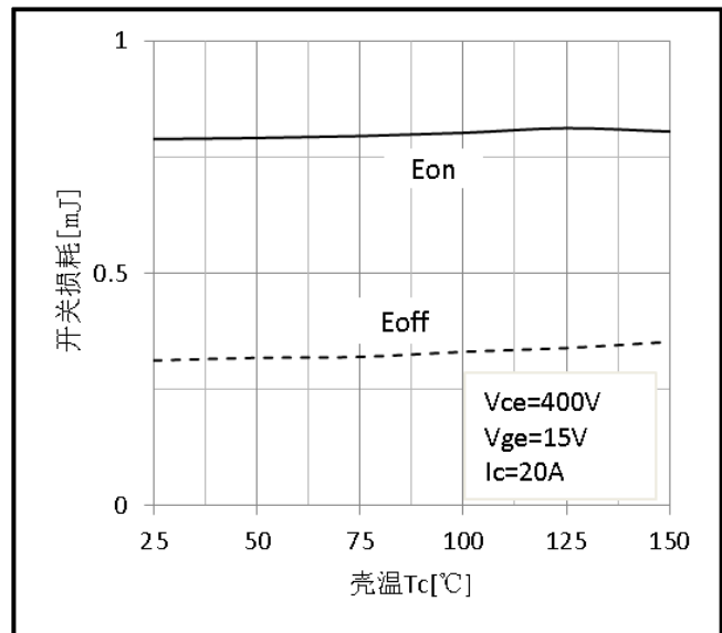
图 10 开关损耗与壳温的关系 (感性负载, 测试电路参考图 E)
