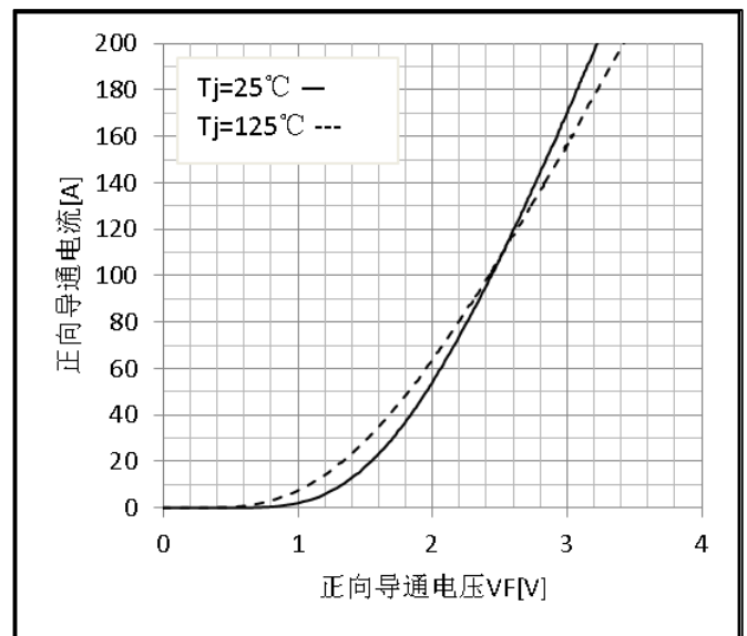
图 16 二极管正向特性
