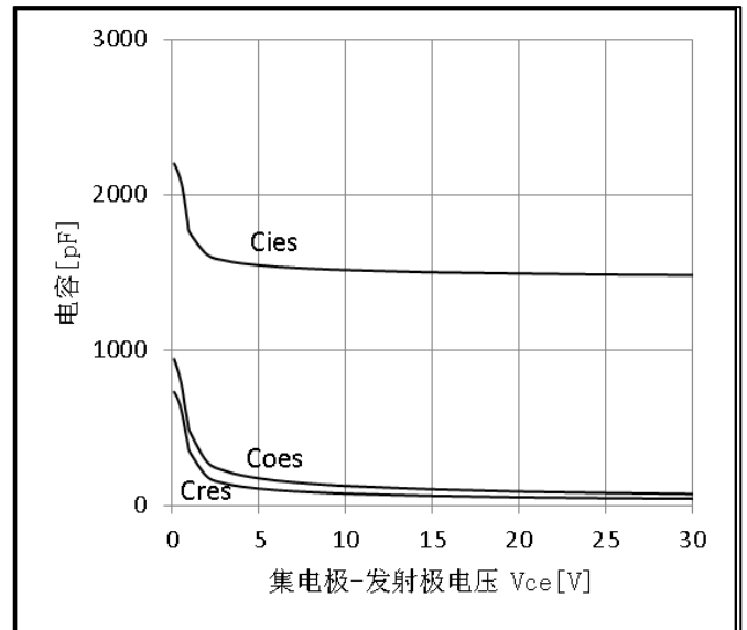
图 14 电容与集电极-发射极电压的关系 ( V_{GE}=0V , f=1MHz )
