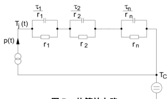
图 D 热等效电路
