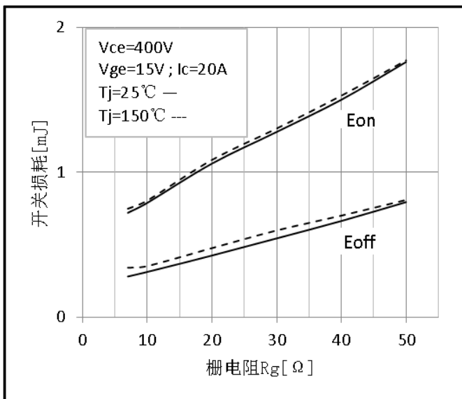
图 7 开关损耗与栅极电阻的关系 (感性负载，测试电路参考图 E)
