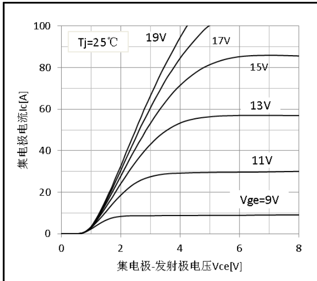
图 1 常温输出特性
