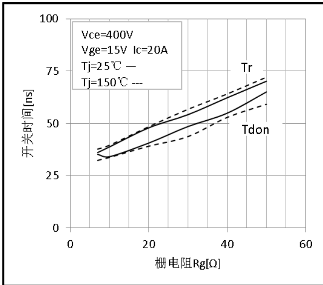
图 5 开通时间与栅极电阻的关系 (感性负载，测试电路参考图 E)
