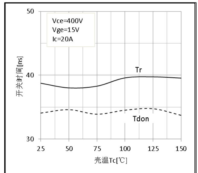
图 8 开通时间与壳温的关系 (感性负载，测试电路参考图 E)
