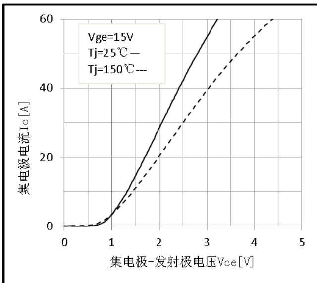
图 3 饱和压降特性
