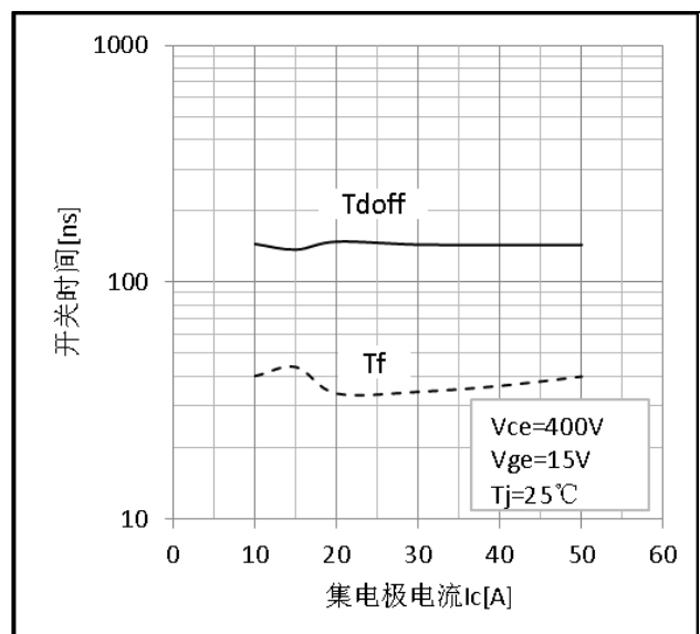
图 12 关断时间与集电极电流的关系 (感性负载, 测试电路参考图 E)
