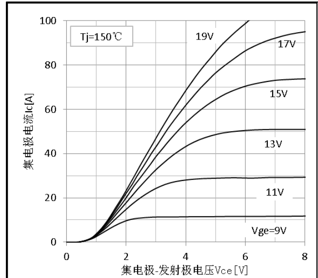
图 2 高温输出特性
