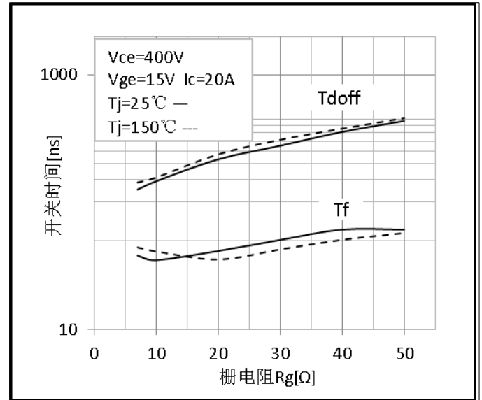
图 6 关断与栅极电阻的关系 (感性负载，测试电路参考图 E)
