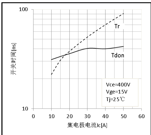
图 11 开通时间与集电极电流的关系 (感性负载, 测试电路参考图 E)
