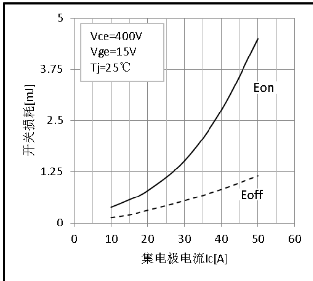
图 13 开关损耗与集电极电流的关系 (感性负载, 测试电路参考图 E)
